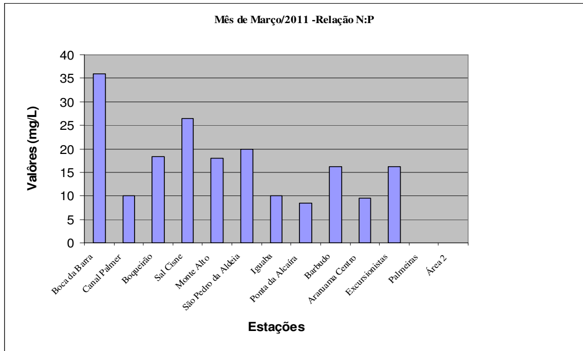
Gráfico 1: Relação entre N/P no mês de março/2011
