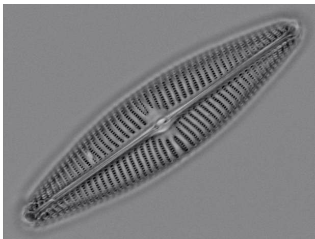
Figura 36- Diatomácea Navicula sp Fonte: http://micro.sakura.ne.jp/bod/hrs_1.htm
